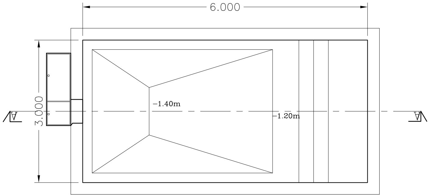
COUPE AA
