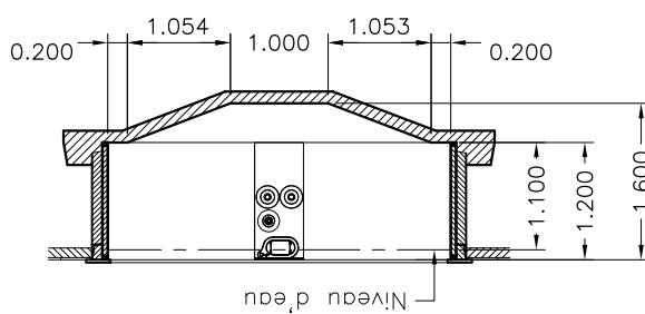
COUPE B-B
